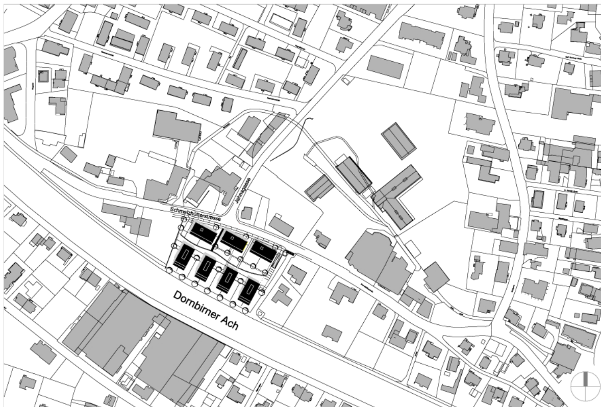
Lageplan
