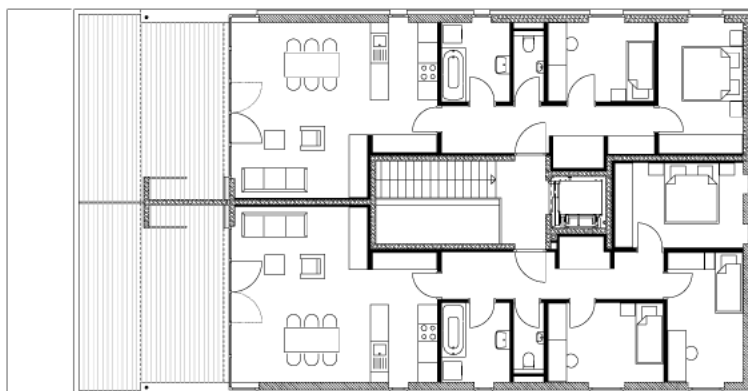
3. Obergeschoss Haustyp 2
