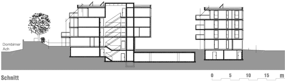
Schnitt
