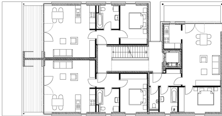
2. Obergeschoss Haustyp 2
